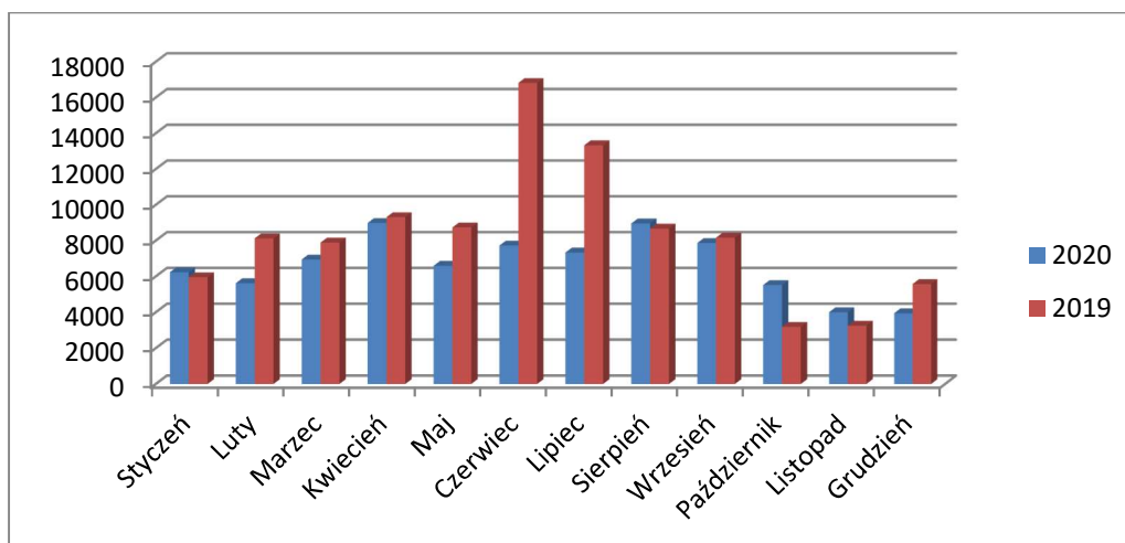
Wykres nr 12. Analiza porównawcza poboru wody w Stacji Uzdatniania Wody w Orlinie
