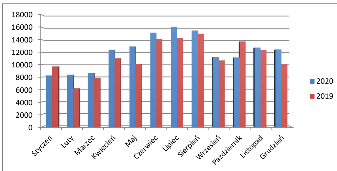
Wykres nr 11. Analiza porównawcza poboru wody w Stacji Uzdatniania Wody w Gizałkach
