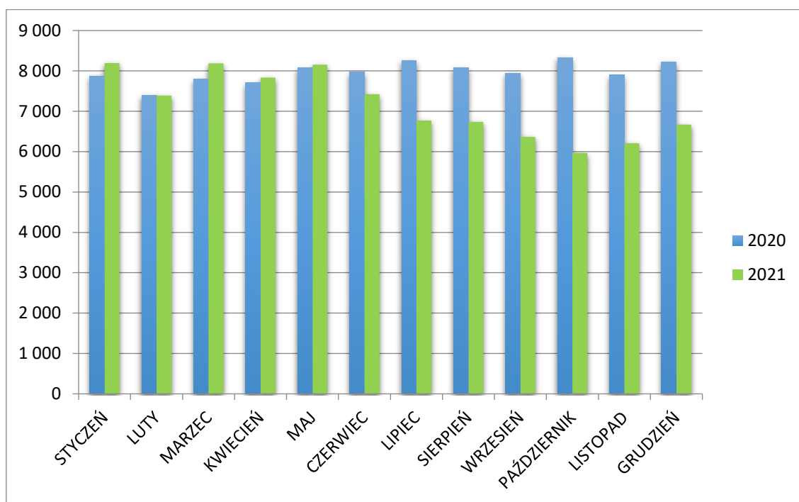
Wykres 14. Ilość przyjętych ścieków Oczyszczalnia Ścieków w Gizałkach w 2021 roku
