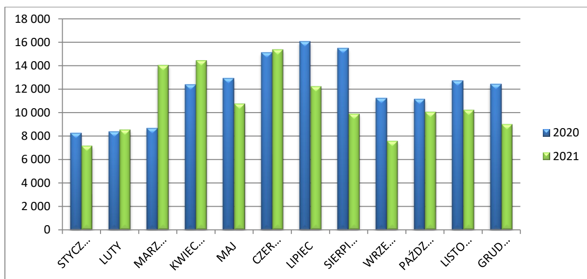
Wykres nr 11. Analiza porównawcza poboru wody w Stacji Uzdatniania Wody w Gizalkach
